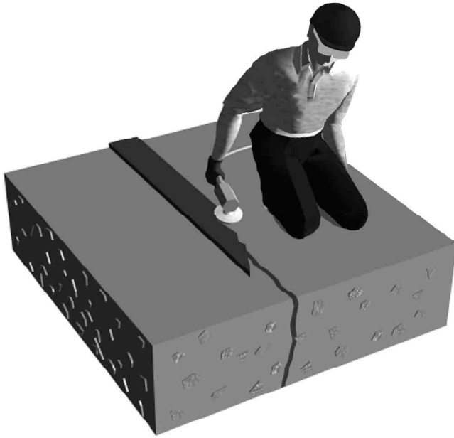
Fig. 6—Remove cap seal.
